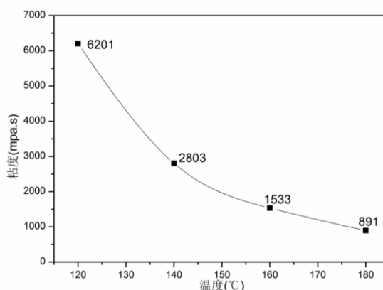
图1、粘度随温度变化曲线图
